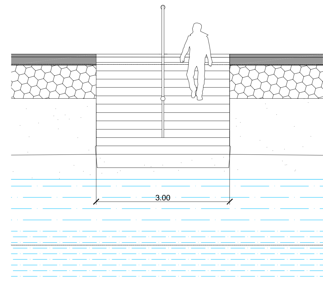
Vooranzicht trap Fluwelensingel, schaal 1:50
