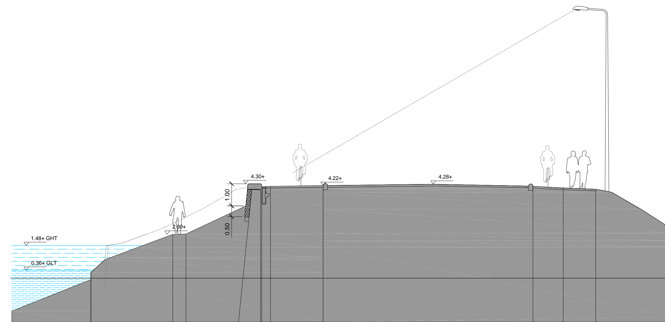
Doorsnede C-C', schaal 1:100
