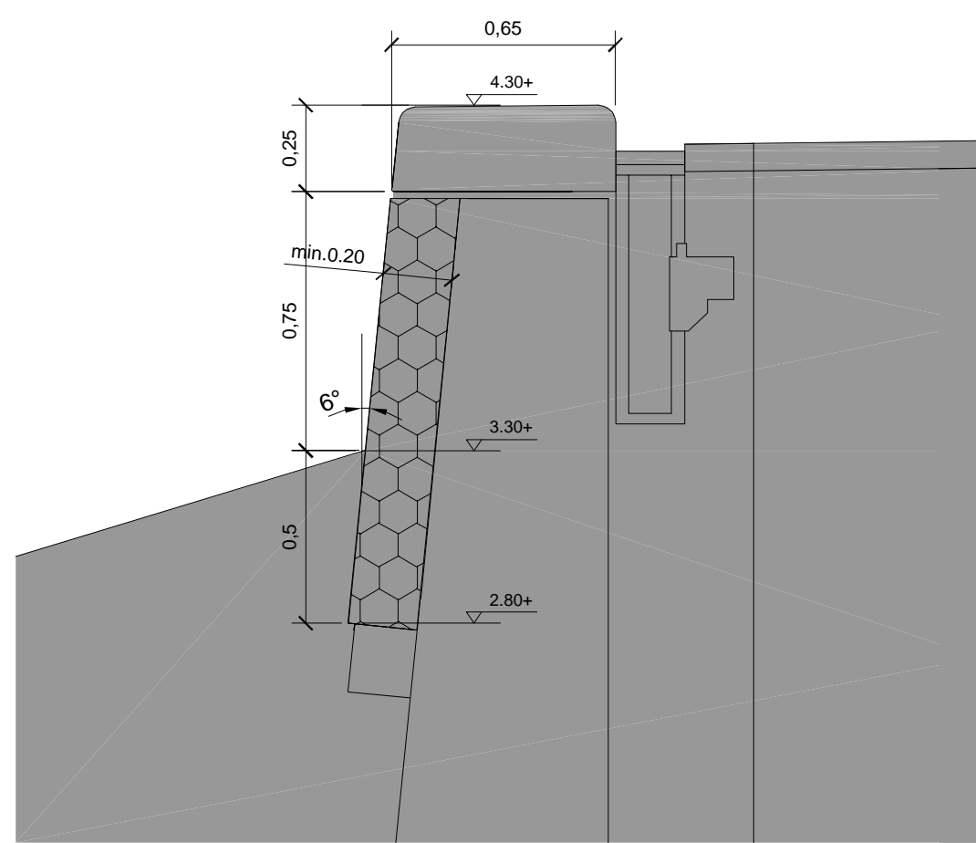
Principe muur, kolk en rabbatstrook, dwarsdoorsnede, schaal 1:20
