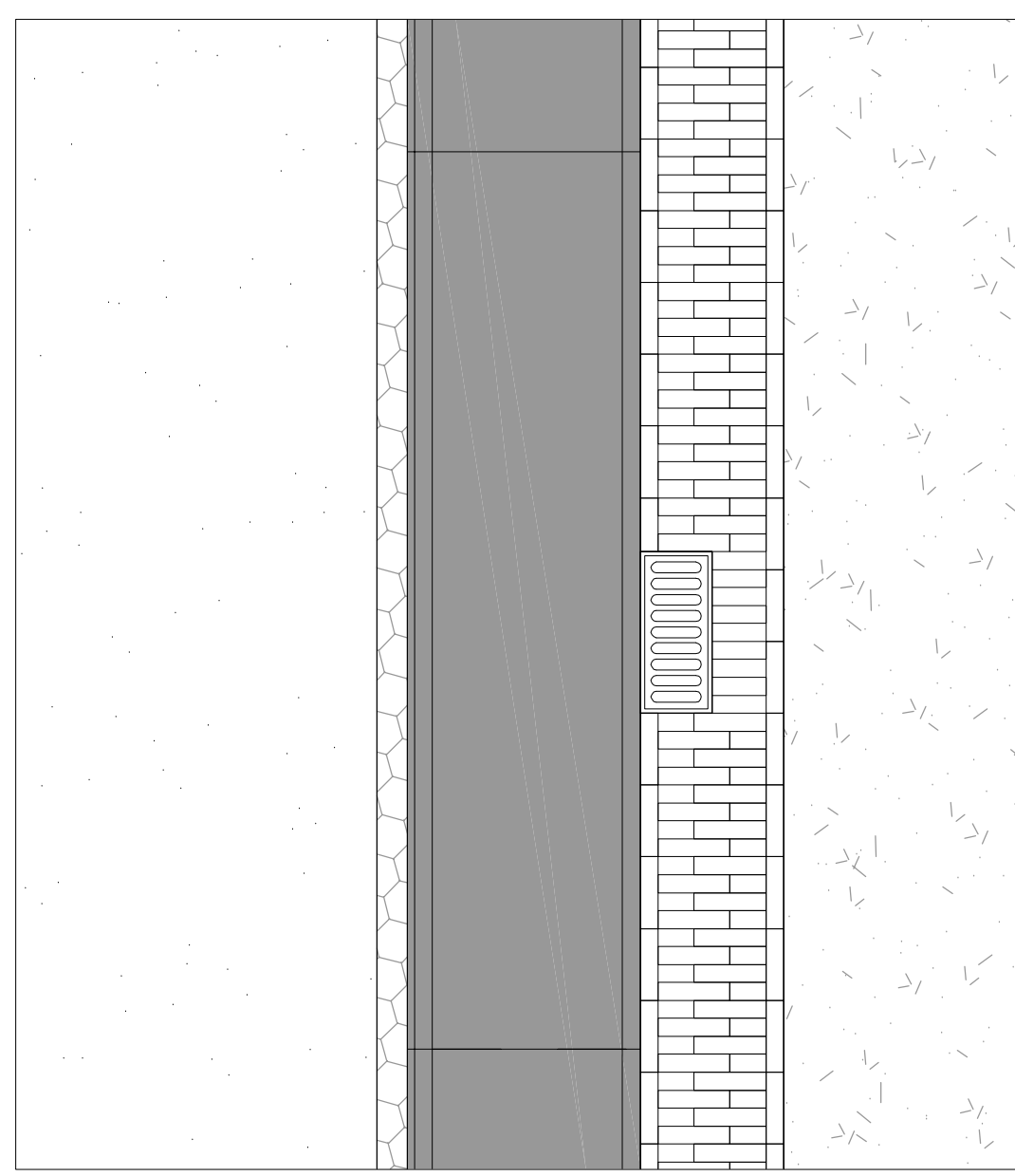
Principe muur, kolk en rabbatstrook, bovenaanzicht, schaal 1:20
