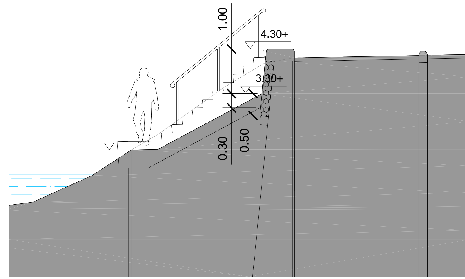
Dwarsdoorsnede trap Fluwelensingel (doorsnede B-B), oprede 188mm, aantrede 230mm, schaal 1:50
