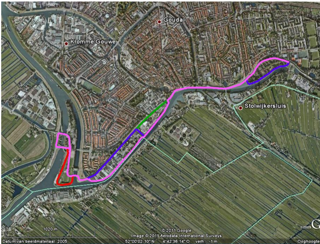
Alternatieven voor dijkverbetering IJsseldijk Gouda
