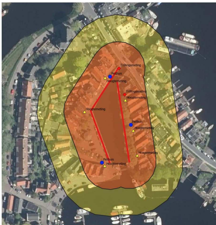
Figuur 1: Overzicht te plaatsen meetpunten en peilbuizen ten behoeve van de nulmetingen.
